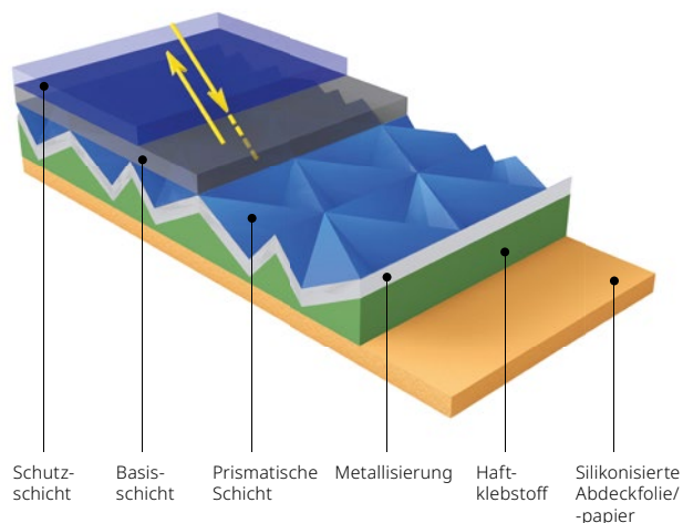
Prismatischer, metallisierter Aufbau Design C
