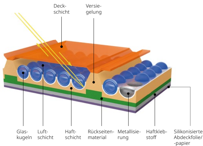
Aufbau mit eingekapselten Glaskugeln Design B
